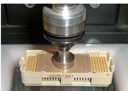
BGA-Kunststoffsocket
