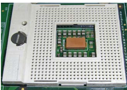
BGA-Prozessorsocket
